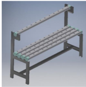
Gambar 2 rangka rak susun media tanam hidroponik
