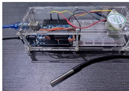
Gambar 9 Hasil rancangan sensor suhu DS18B20
