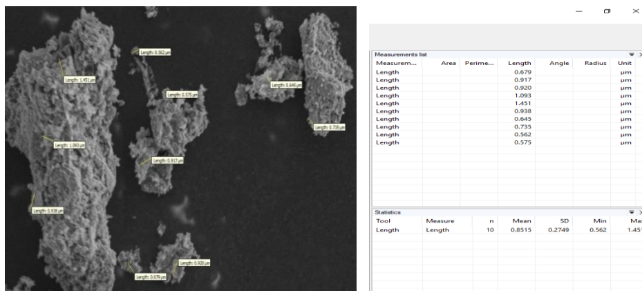
Gambar 1. Sampel A hasil SEM bata merah yang dianalisis dengan software digimizer [1]
