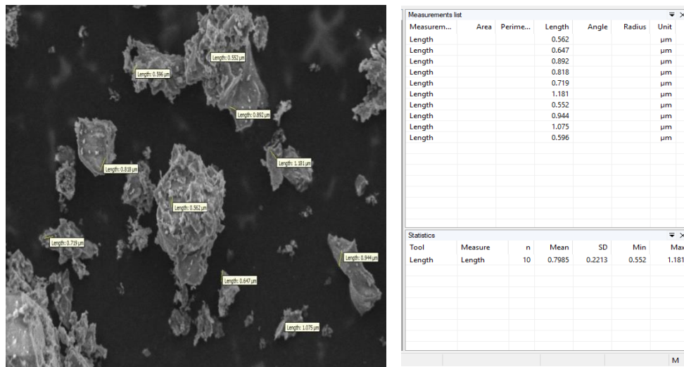
Gambar 3. Sampel C hasil SEM bata merah yang dianalisis dengan software digimizer [3]
