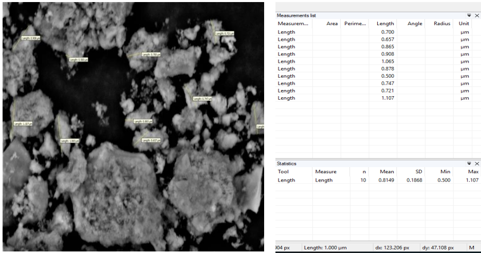
Gambar 2. Sampel B hasil SEM bata merah yang dianalisis dengan software digimizer [2]
