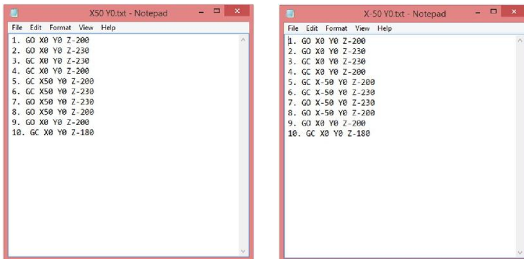
Gambar 14. Tahapan untuk posisi peletakan (a) (50,0) mm (b) (-50,0) mm.
