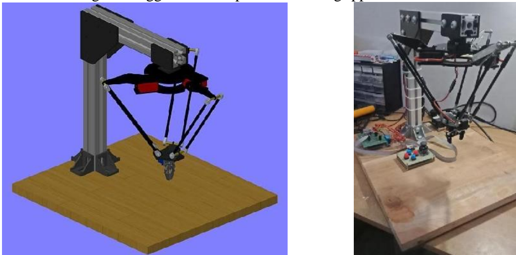
Gambar 2. Desain mekanik keseluruhan robot delta.
