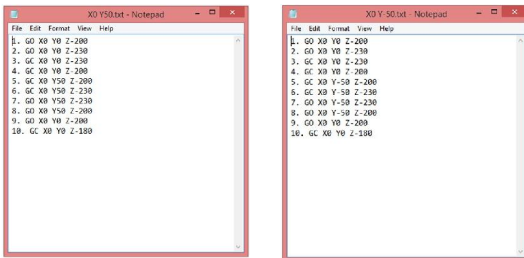
Gambar 15. Tahapan untuk posisi peletakan (a) (0,50) mm (b) (0,-50) mm.
