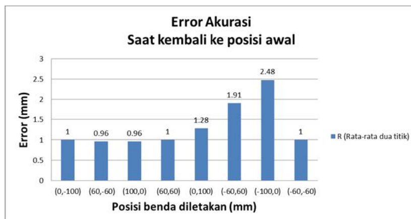
Gambar 12. Grafik error akurasi saat kembali ke posisi awal.
