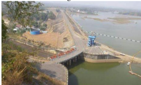
Gambar 2. Bendungan Karian
