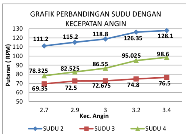
Gambar 4. Grafik perbandingan sudu dan kecepatan
