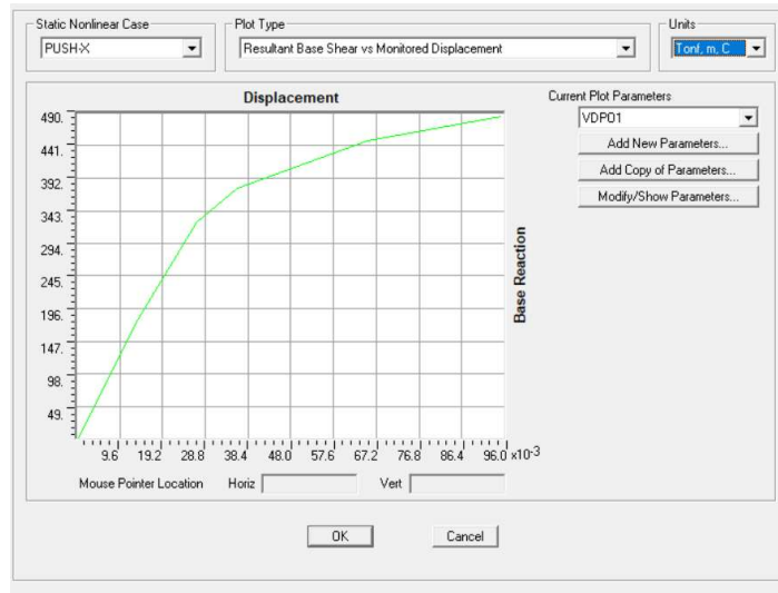
Gambar 2. Kurva Kapasitas Arah x (PUSHX) Sumber : Program Komputer
