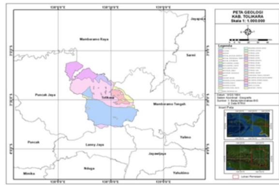
Gambar 4. Peta Geologi Kabupaten Tolikara
